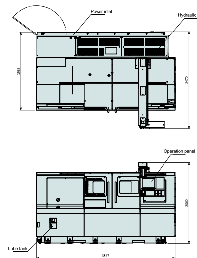
GENOS L3000-e (Lx1100/Mx1000)
