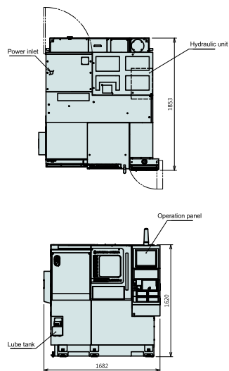
GENOS L2000-e (Lx290)
