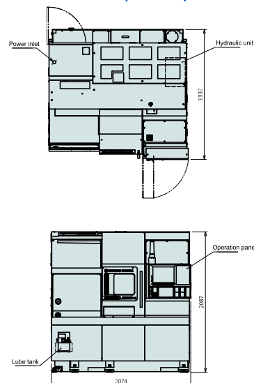
GENOS L2000-e (MYx380)
