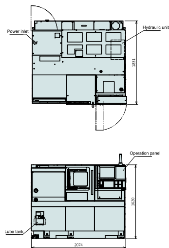
GENOS L2000-e (MYx380)
