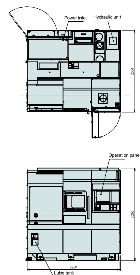
GENOS L3000-e (MYx400)
