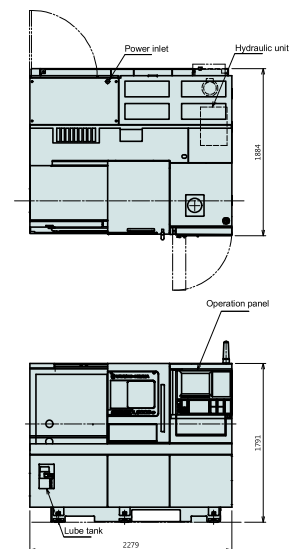
GENOS L3000-e (Lx500/Mx450)
